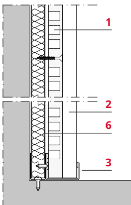
FINITURA INFERIORE LOWER FINISHING
