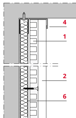
FINITURA SUPERIORE UPPER FINISHING
